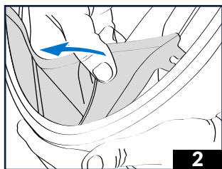
2 - Retourner le casque et défaire chacune des joues, une après l'autre.
